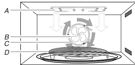
A. Élément de cuisson au grill B. Ventilateur de convection C. Élément de convection D. Grille de convection
